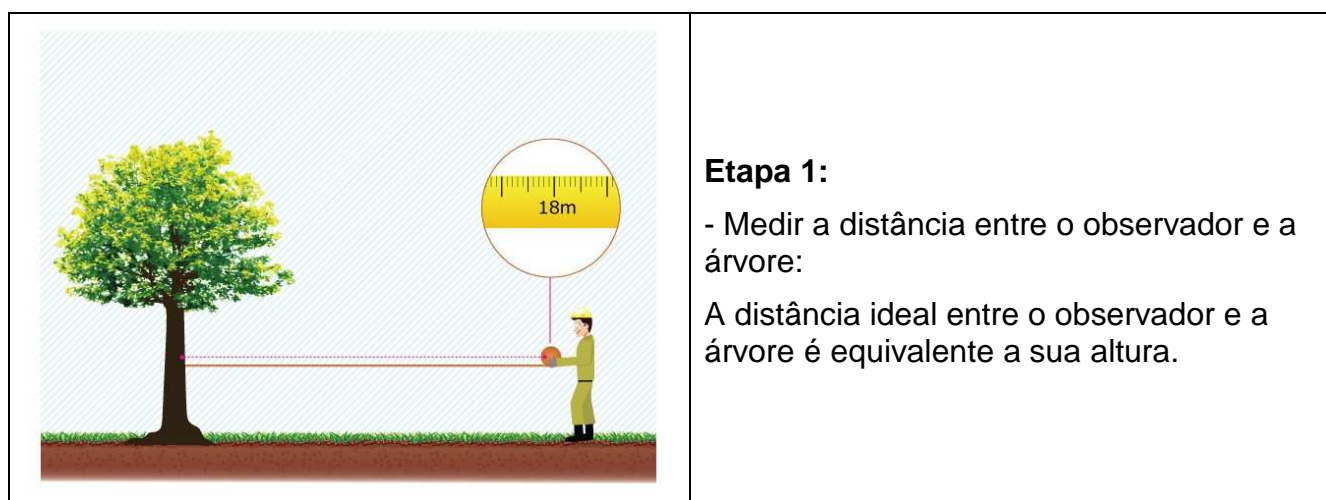
Figura 35: Etapa 1 da medição de altura com Clinômetro
