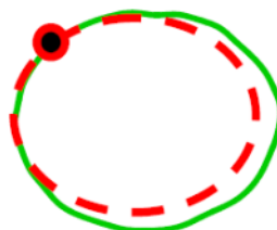
Figura 42: Datum Local com referência na zona de interesse
