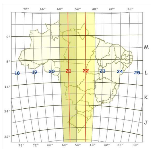
Figura 45: Projeção do Meridiano Central dos Fusos 21 e 22.
