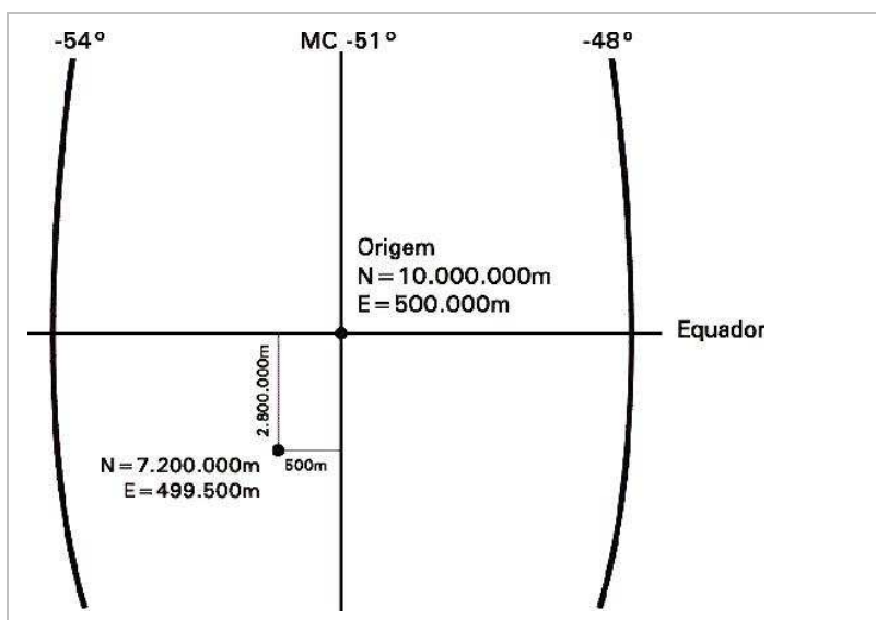
Figura 47: Sistema cartesiano métrico de referência com origem no centro do fuso.
