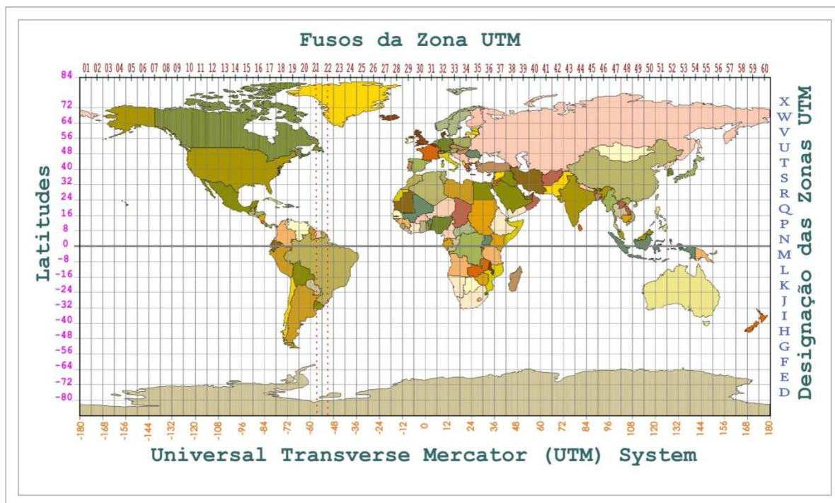
Figura 44: Terra projetada no Sistema de Projeção Universal Transversa de Mercator.
