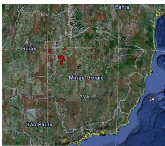
Figura 46: Detalhe do Fuso 23 K – com pontos seleccionados para o teste do IFN
