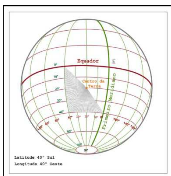
Figura 43: Sistema de coordenadas cartesiano e curvilíneo.
