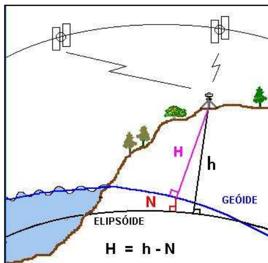
Figura 40: Diferentes representações da superfície terrestre.
